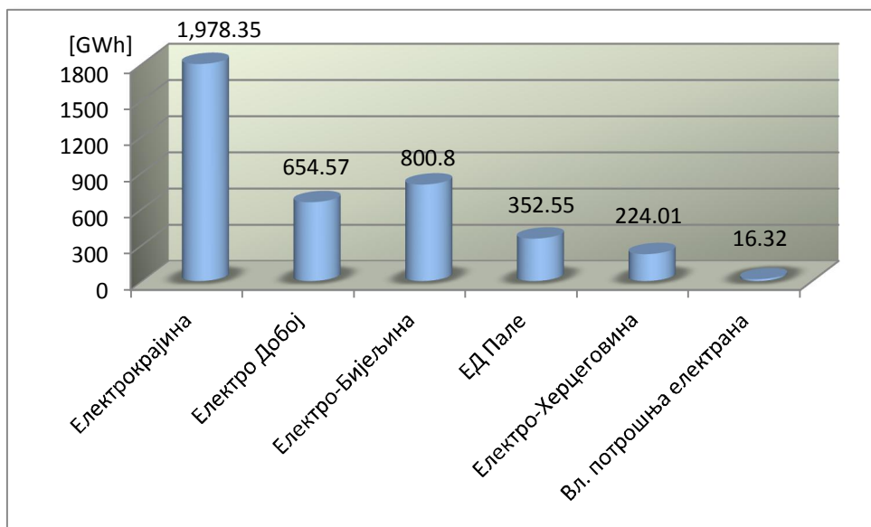
Сл. 2.7 Биланс укупне потрошње електричне енергије за 2017. г.
