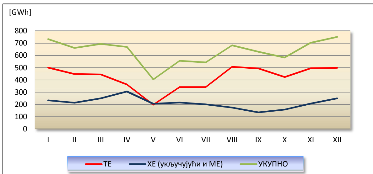
Сл. 2.2 План производње електричне енергије у 2017. години
