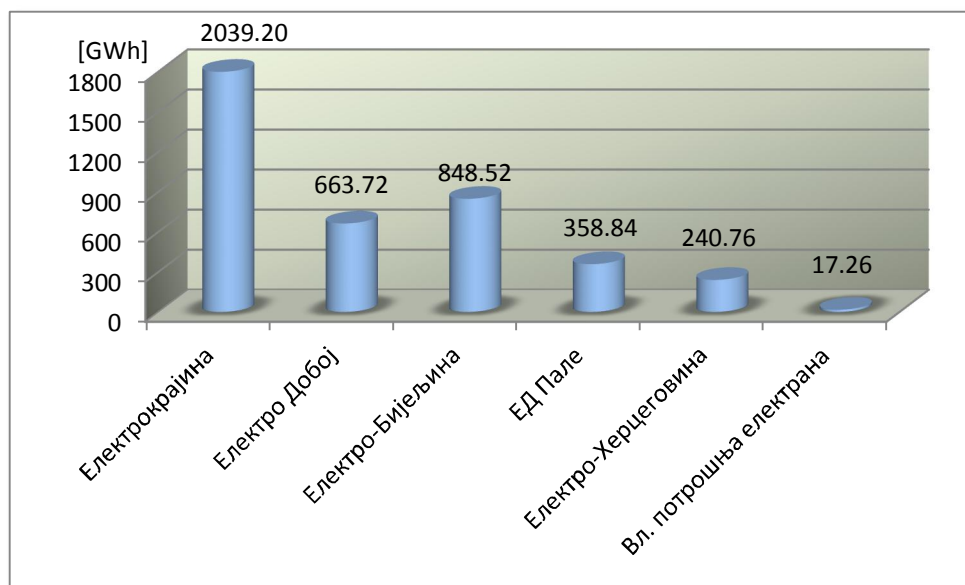
Сл. 1.10 Биланс укупне потрошње електричне енергије за 2019. г.
