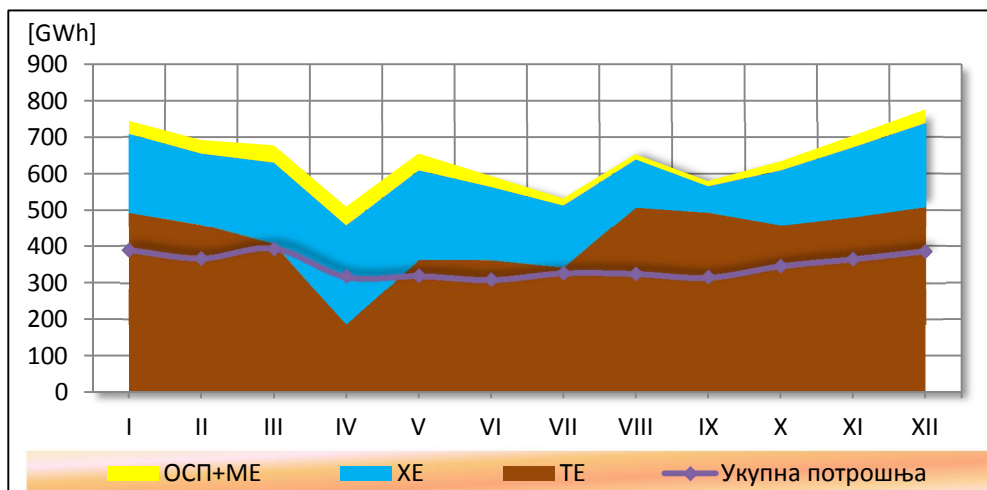
Сл. 1.13 Структура укупне производње и укупне потрошње електричне енергије у Републици Српској у 2019. години по мјесецима
