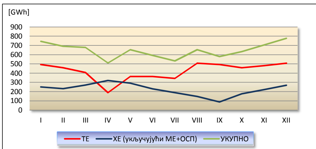
Сл. 1.3 План производње електричне енергије по мјесецима у 2019. години
