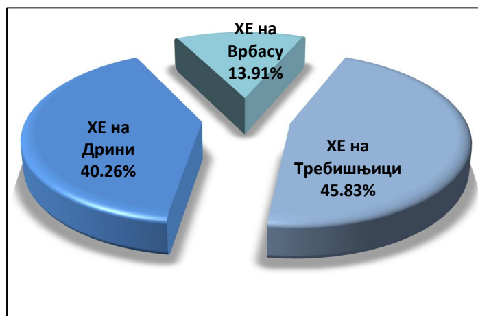
Сл. 1.7 Учешће појединих ХЕ у укупно планираној производњи ел. енергије из хидроелектрана у 2019. години
