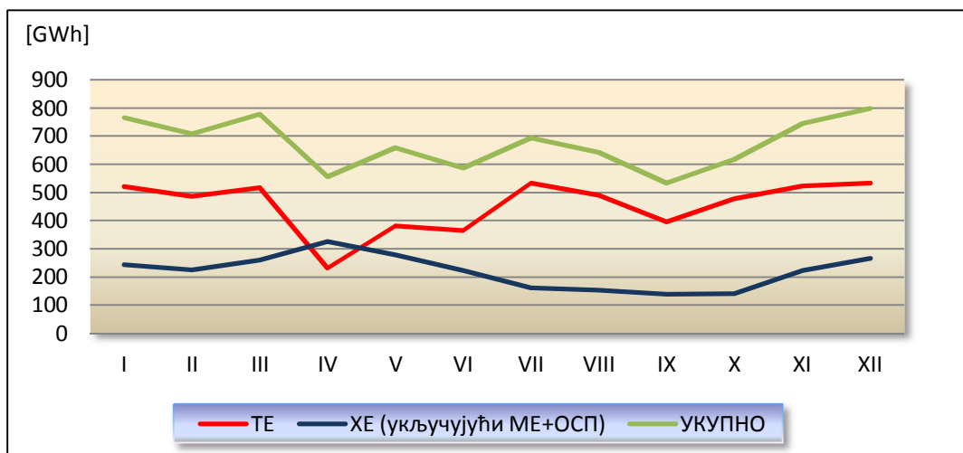
Сл. 1.3 План производње електричне енергије по мјесецима у 2018. години
