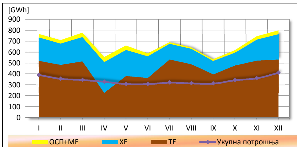
Сл. 1.13 Структура укупне производње и укупне потрошње електричне енергије у Републици Српској у 2018. години по мјесецима
