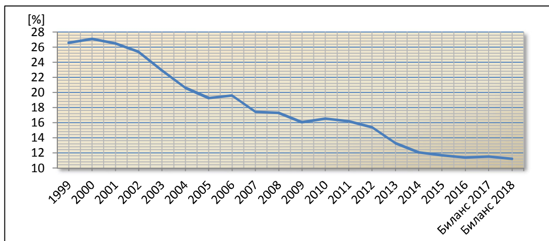
Сл. 1.12 Тренд укупних дистрибутивних губитака
