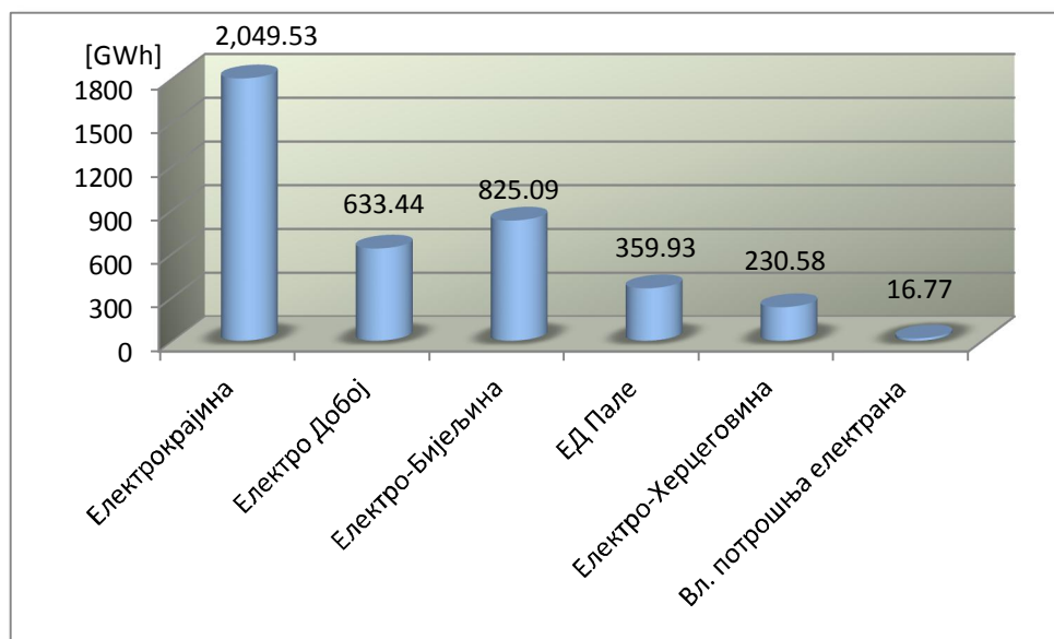
Сл. 1.10 Биланс укупне потрошње електричне енергије за 2018. г.
