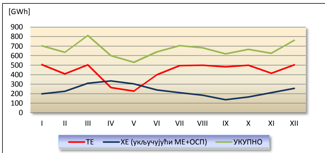
Сл. 1.3 План производње електричне енергије по мјесецима у 2020. години
