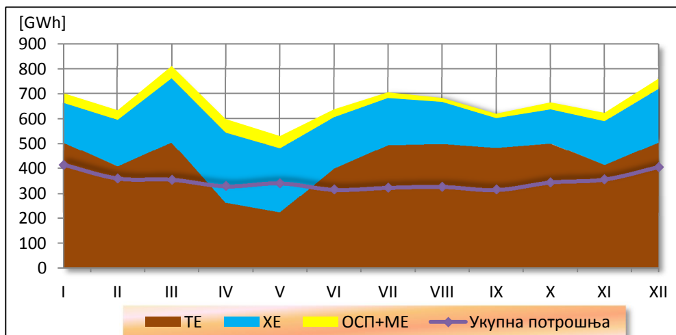
Сл. 1.14 Структура укупне производње и укупне потрошње електричне енергије у Републици Српској у 2020. години по мјесецима
