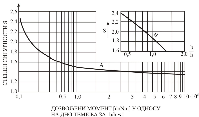
Слика 4. Дијаграм за прорачун темелја према методи Клајнлогел - Бирклина
