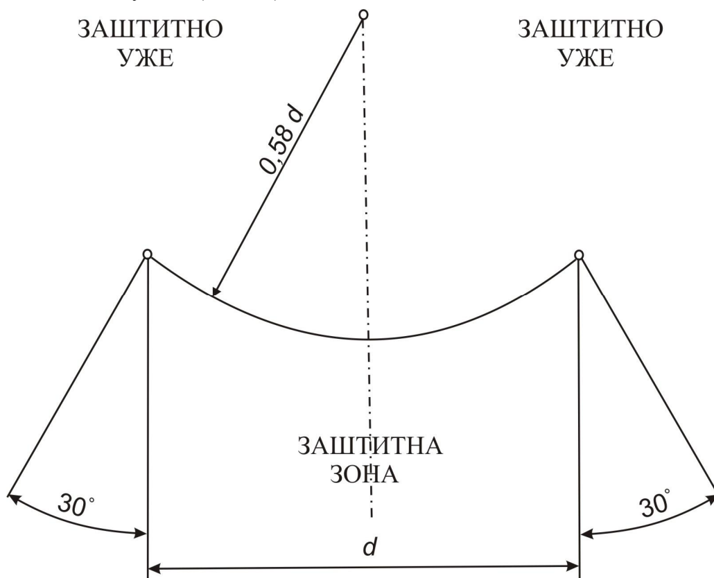
Слика 2. Заштитно уже и заштитна зона
