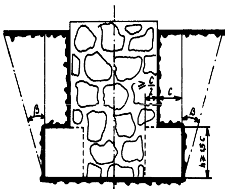
Слика 5. Бетонски темељ укопан у тло
